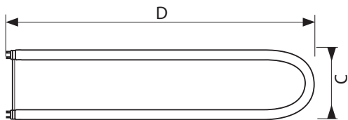
FB32T8/6 TL735 ALTO
